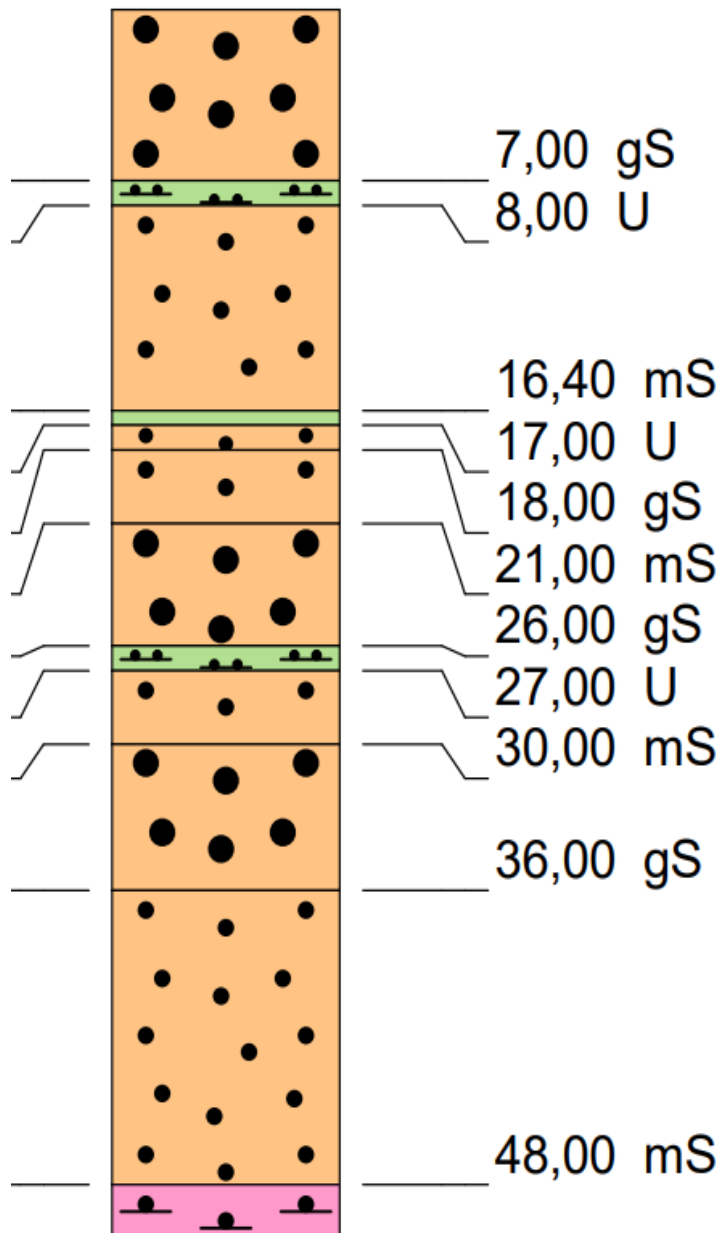
Abb. 1: Vorprofil GWM Bremsdorf 1/26
